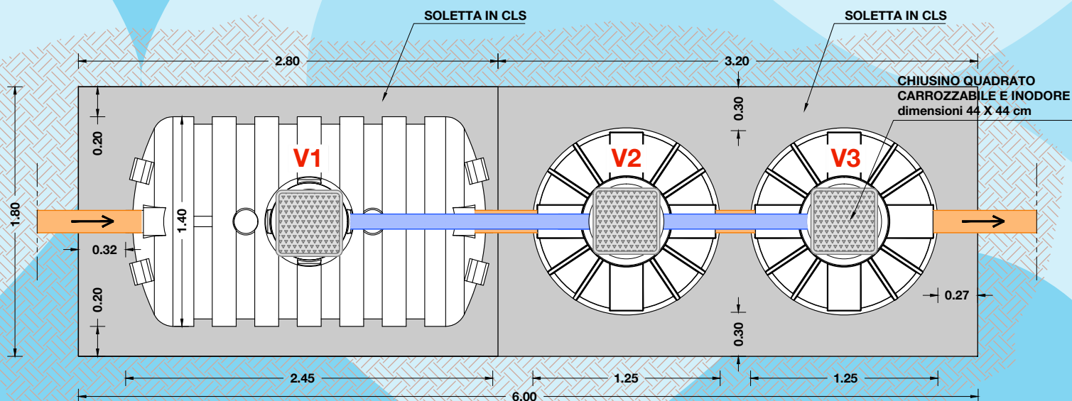
VISTA IN PIANTA
