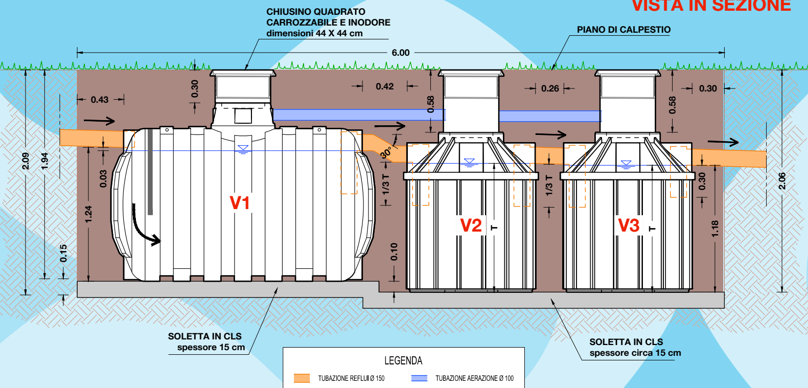
VISTA IN SEZIONE
