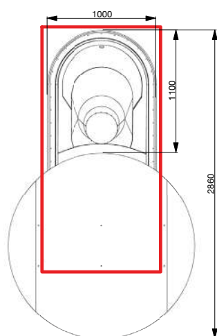
VISTA DALL'ALTO
