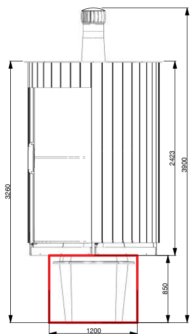
VISTA FRONTALE
