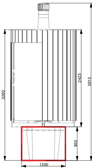
FRONTANSICHT ANSICHT
