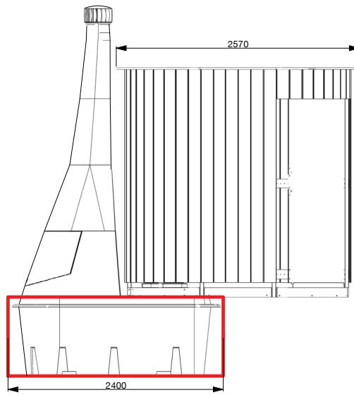
SEITENANSICHT
